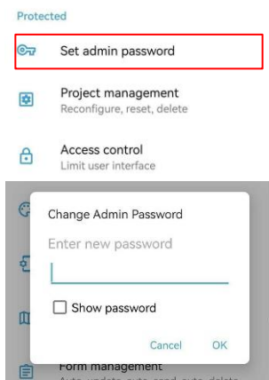
Figura 19: Senha de administração
