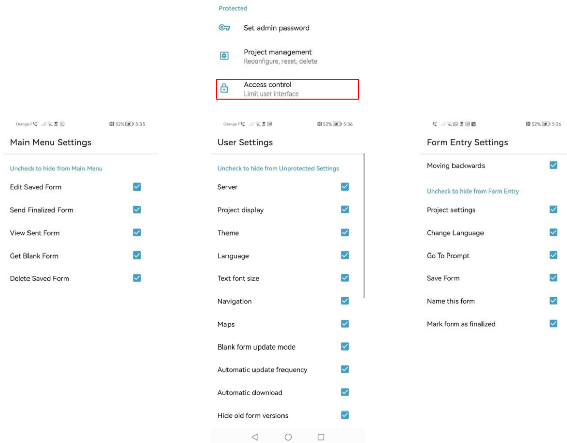
Figura 18: Botões de ocultação
