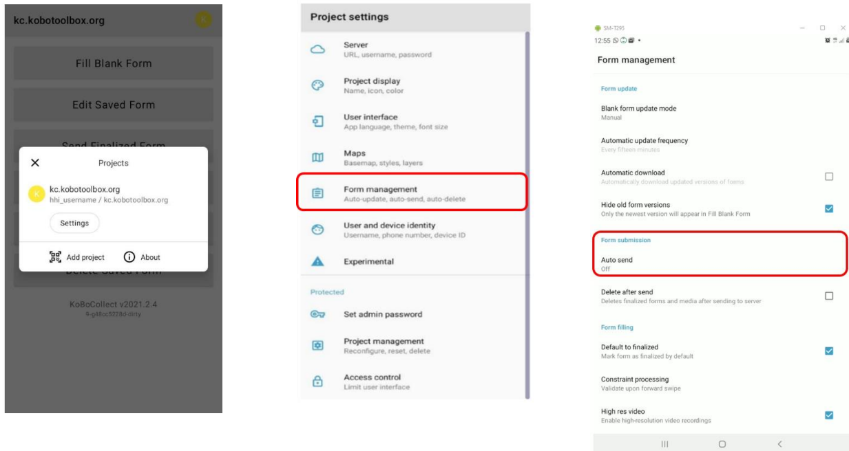
Figura 15: funções para desativar envio automático
