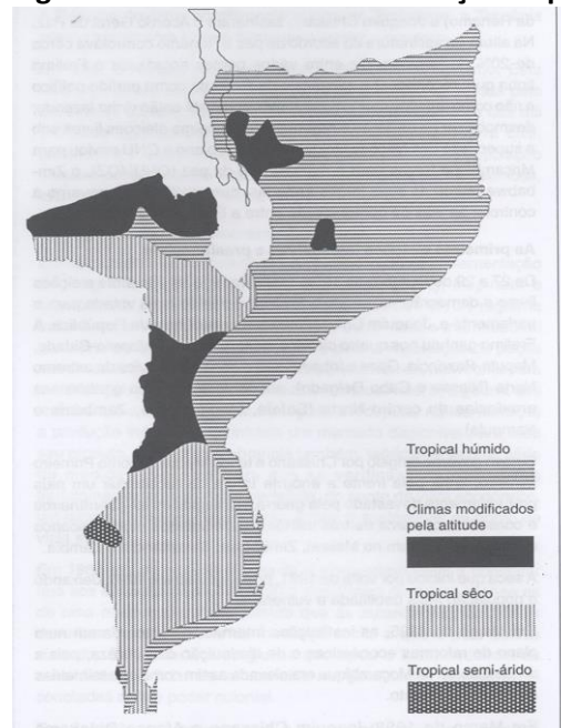
Figura 1: Zonas Climáticas de Moçambique
